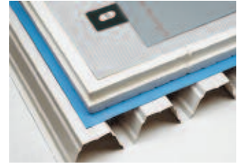
Çıt çitli sistemi ile mekanik sabitleme
